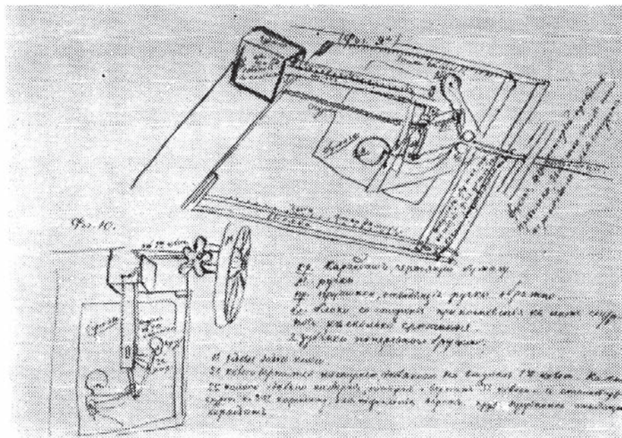
Чертеж путеграфа священника Дернава.
